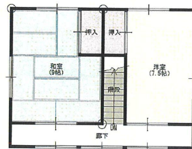
2階 平面図
