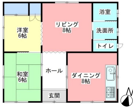
▲間取図
