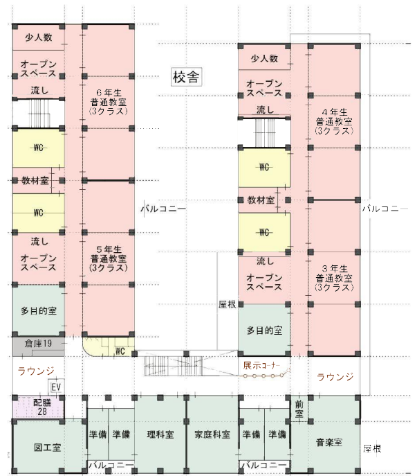
↓ 2階平面図
