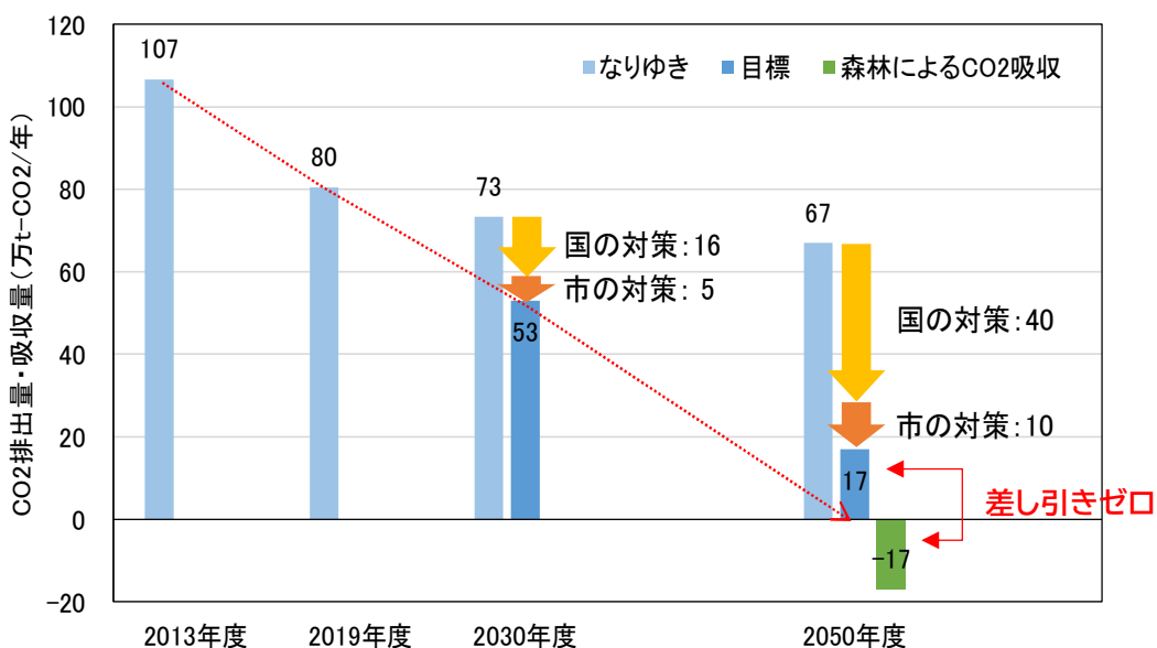
図 4.1 CO 2 排出量削減シナリオ
