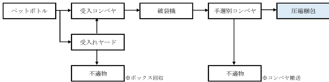
図 6-4 ペットボトル処理基本フロー
