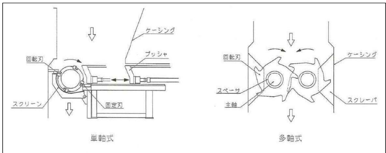
図 7-2-1 低速回転破碎機（単軸式と多軸式）
