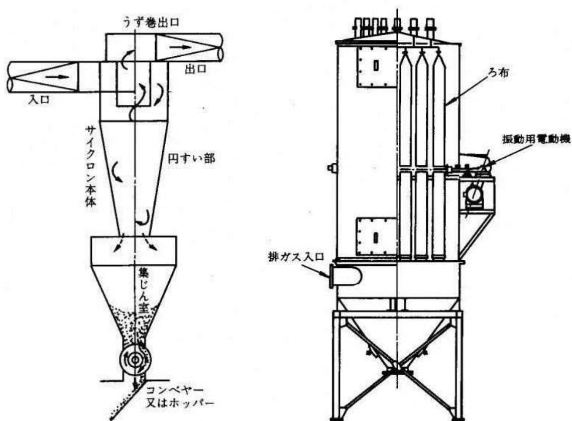
図 7-7-1 (左) サイクロン方式、(右) ろ過式集じん方式
