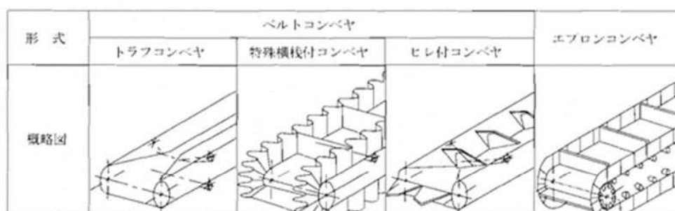
図 7-3-1 搬送設備
