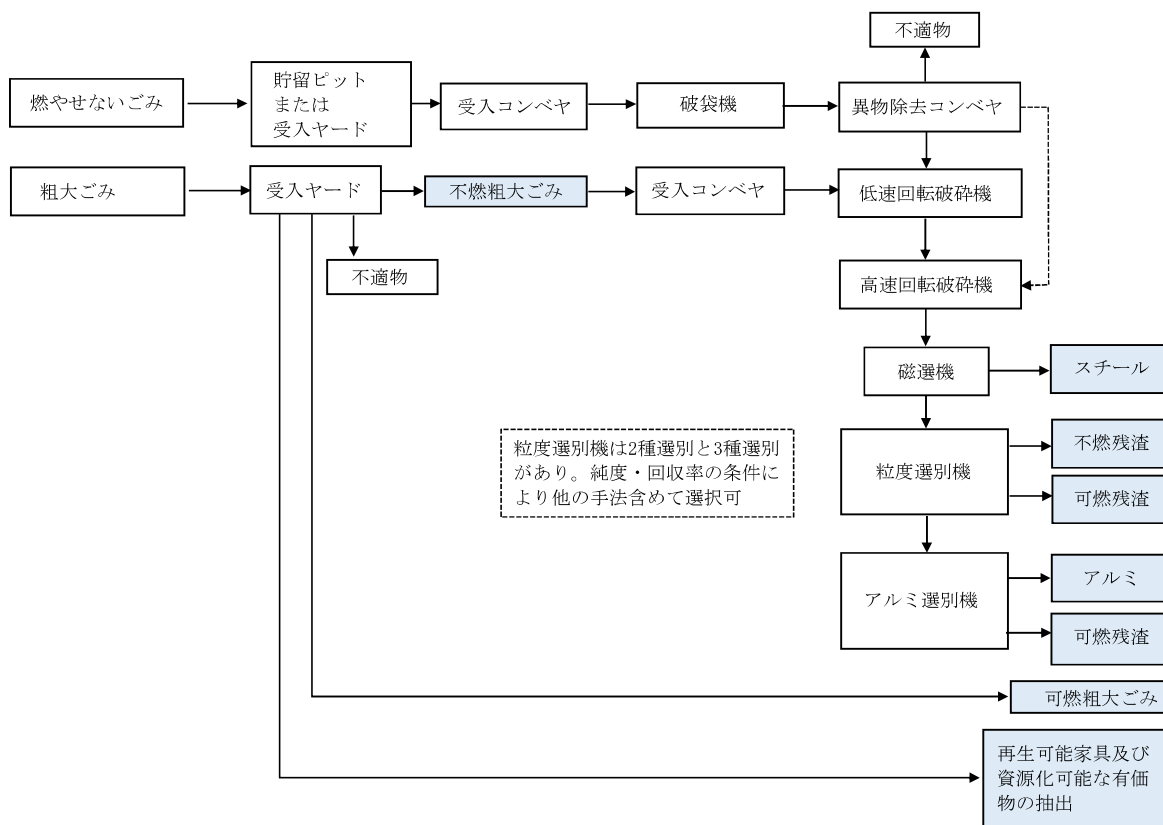
図 6-1 燃やせないごみ・不燃粗大ごみ処理基本フロー
