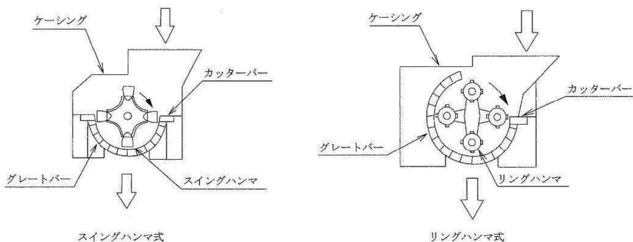
図 7-2-4 横型高速回転破砕機（スイングハンマ式とリングハンマ式）
