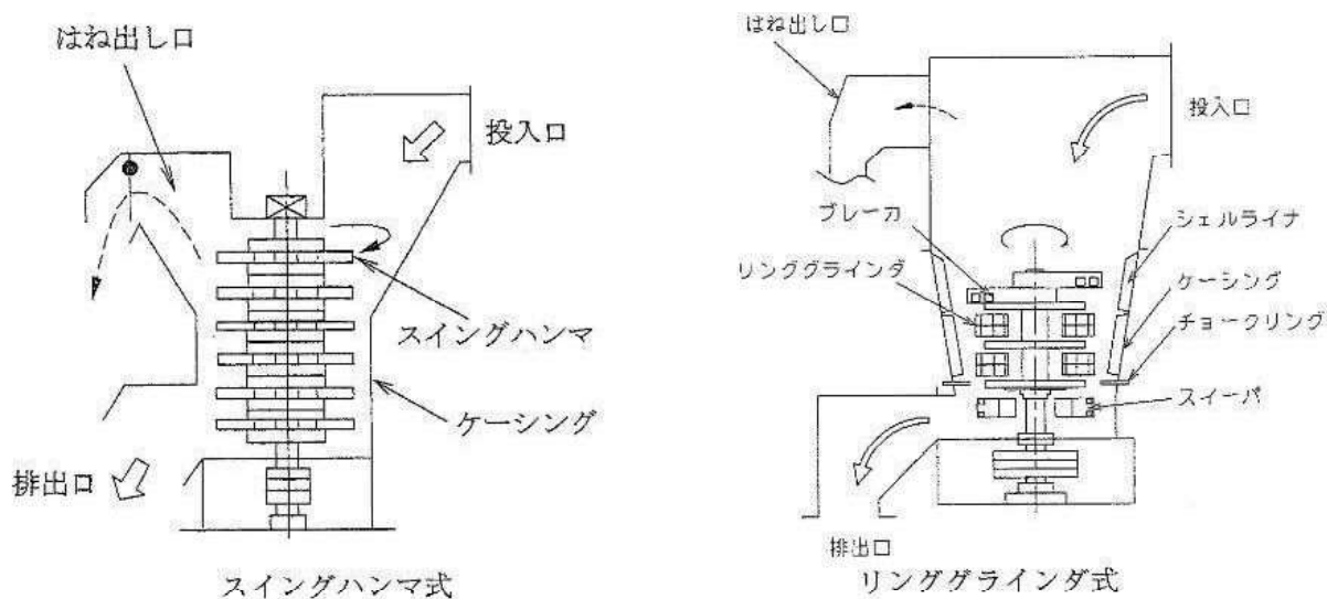
図 7-2-3 縦型高速回転破砕機（スイングハンマ式とリンググラインダ式）
