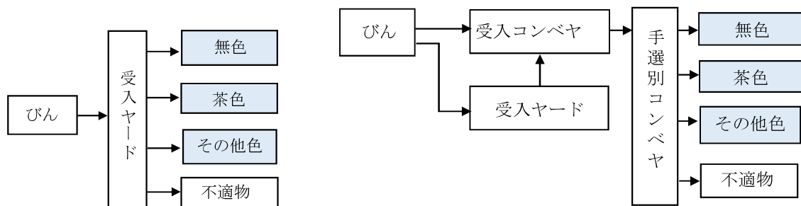
図 6-2 びん処理基本フロー（ヤード手選別とコンベヤ手選別）
