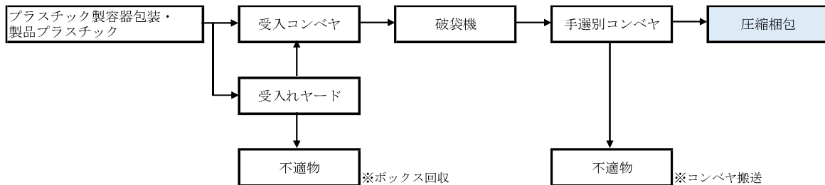
図 6-5 プラスチック製容器包装・製品プラスチック処理基本フロー
