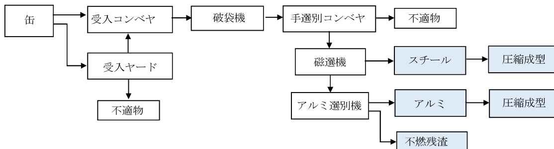
図 6-3 缶処理基本フロー
