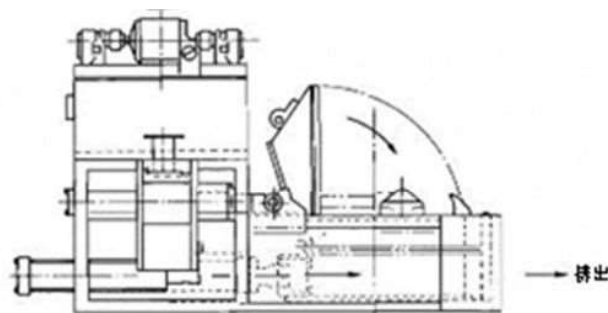
図 7-5-1 油圧二方締め式圧縮成型機
