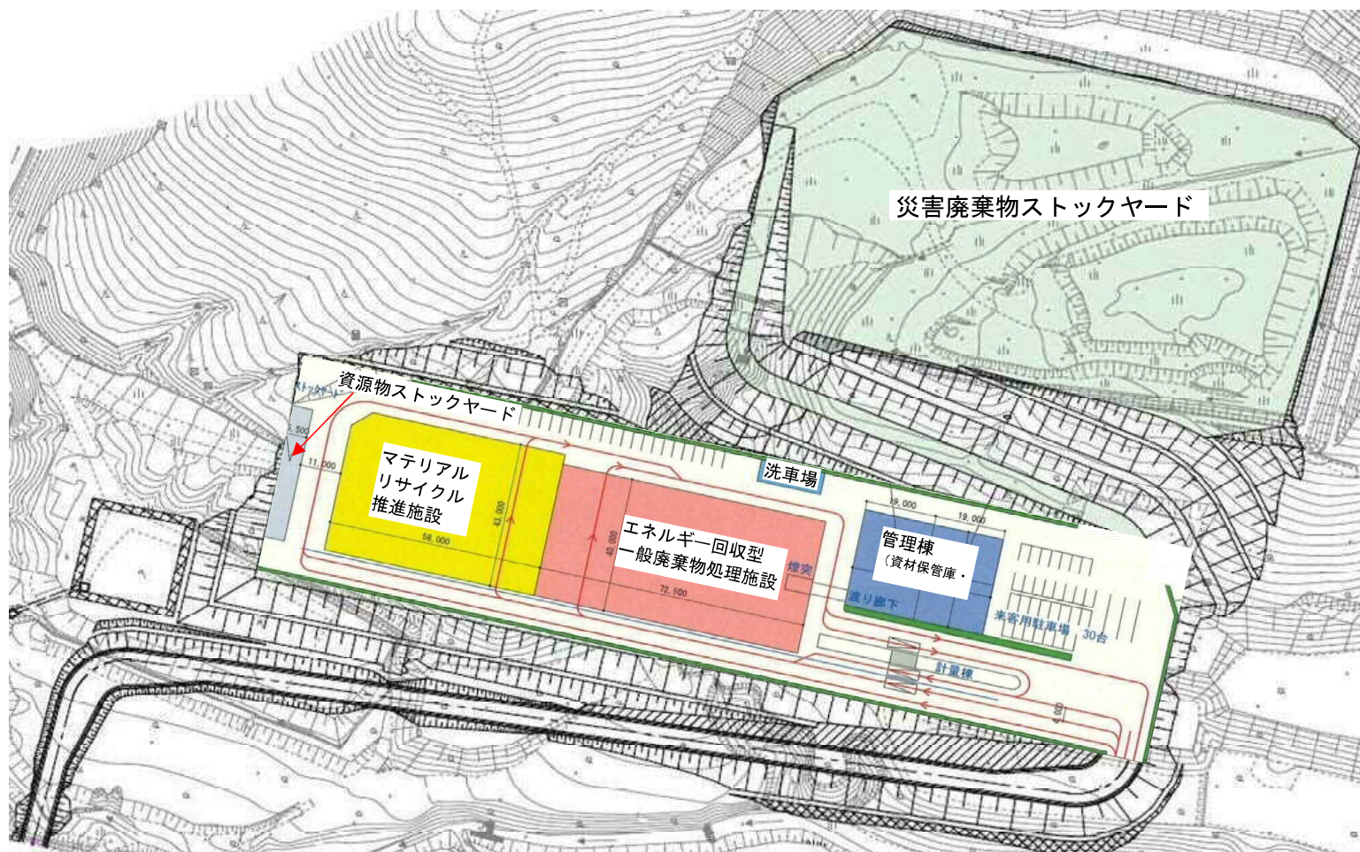
図 10-1-1 全体配置図
