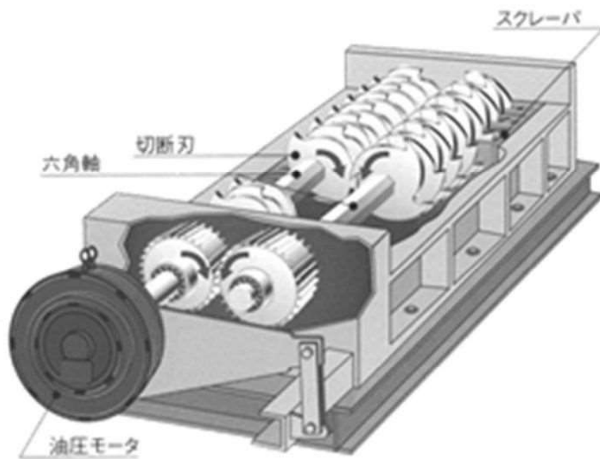
図 7-2-2 低速回転破碎機（多軸式）の例
