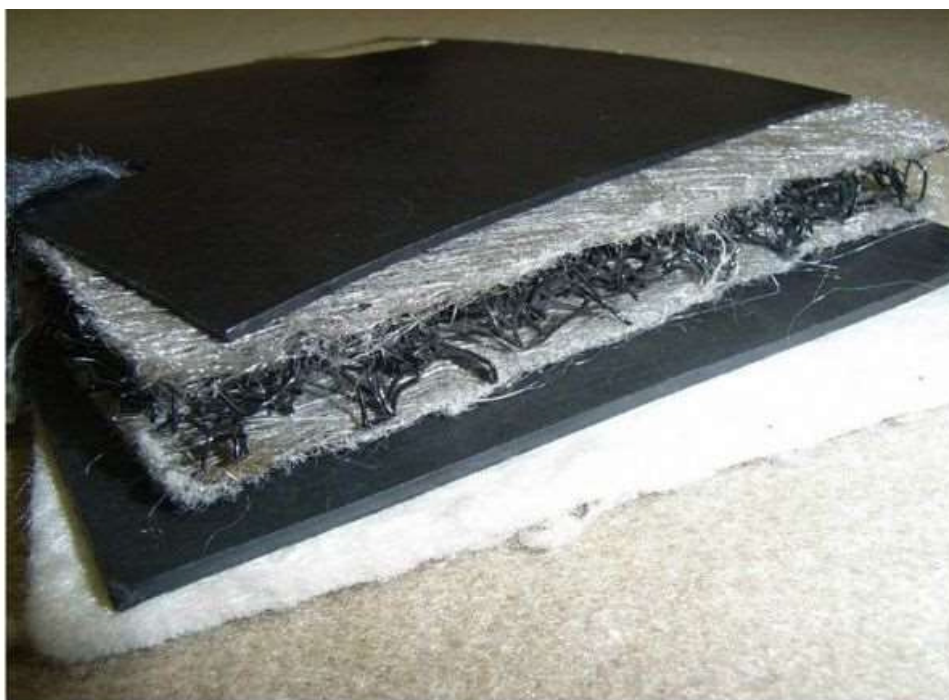
二重しゃ水シートの構造例
