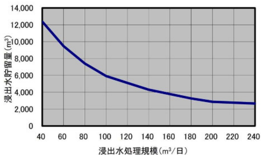
図3-6-9 浸出水処理施設規模と必要調整槽容量の関係（1998年）
