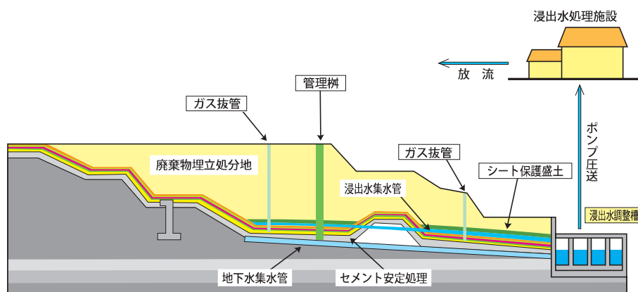
フローシート
