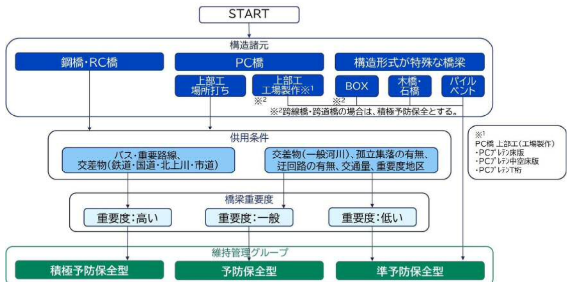
図-3.3 維持管理グループ選定フロー
