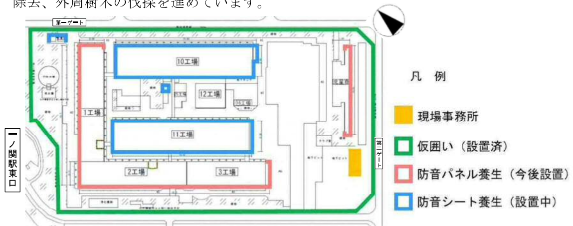
【全体平面図】
