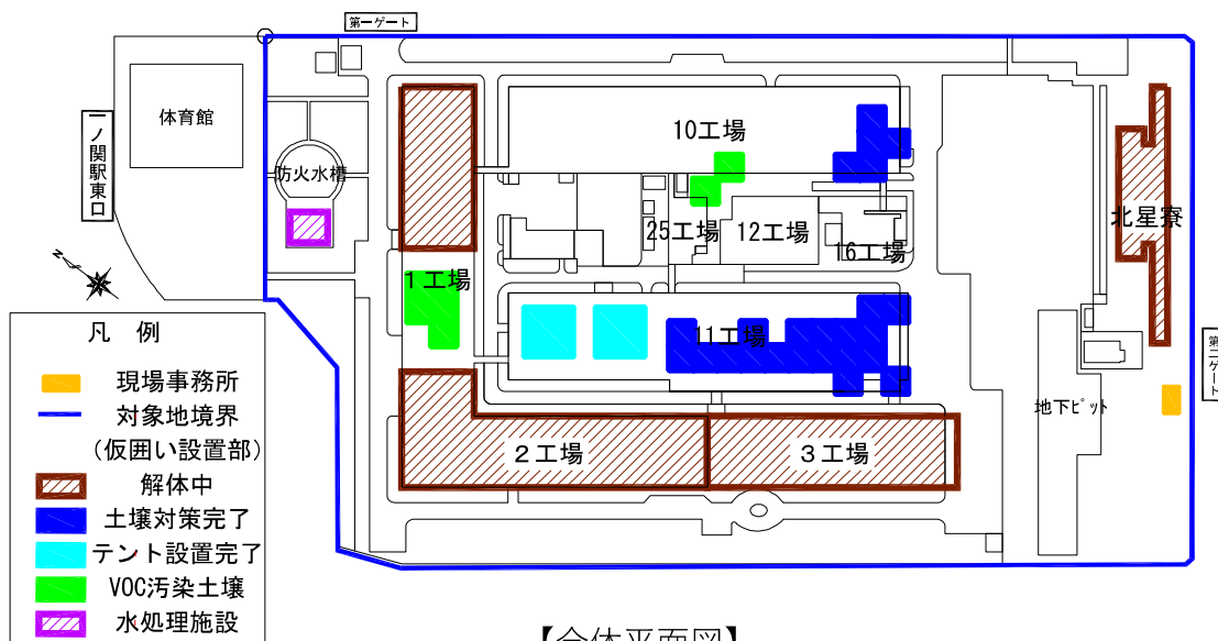
【全体平面図】
